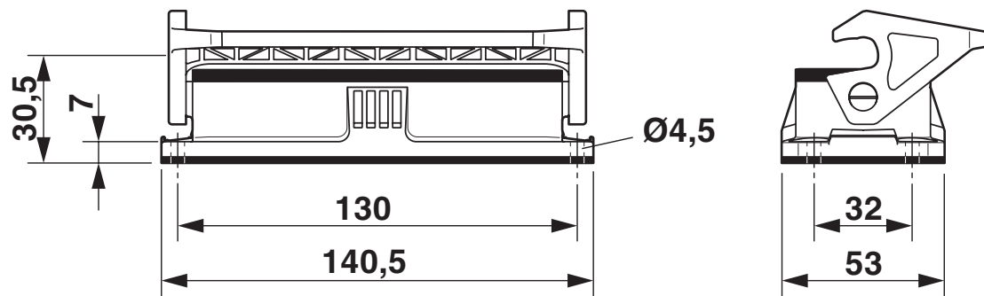
尺寸图
