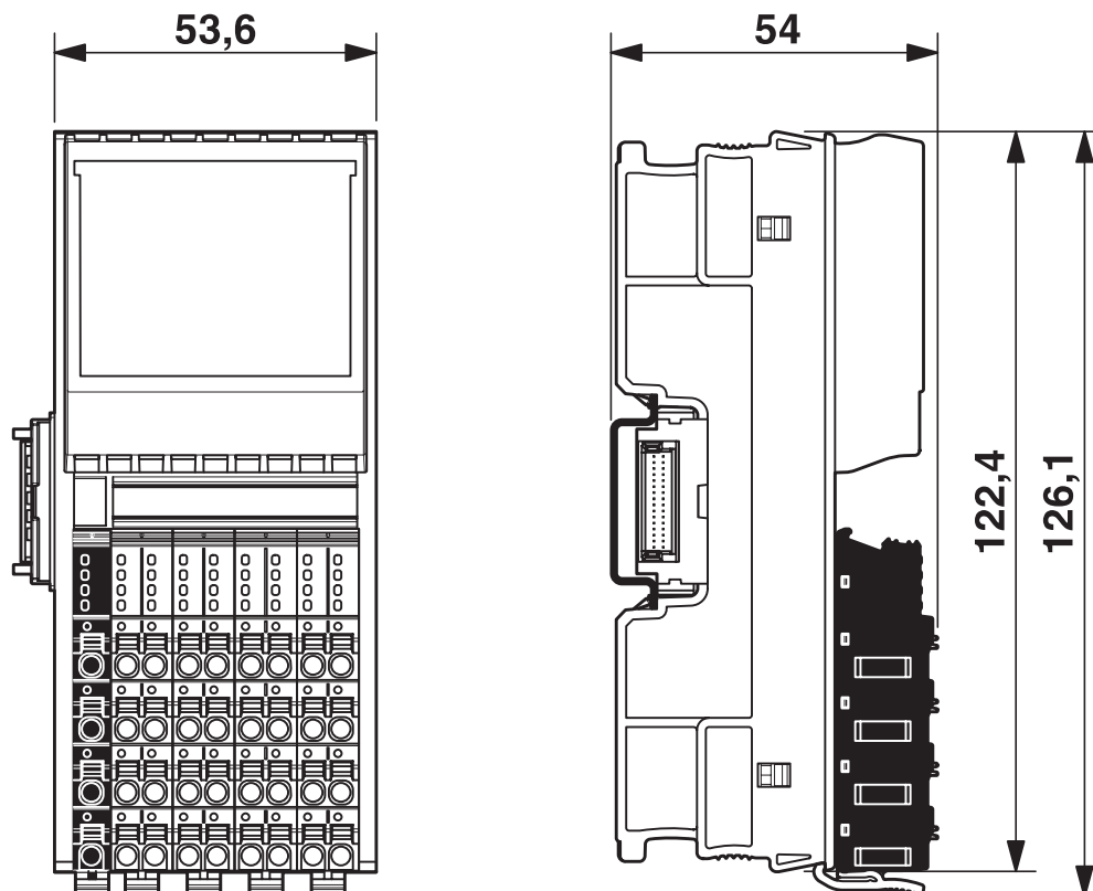
尺寸图
