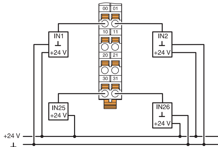
接线图
