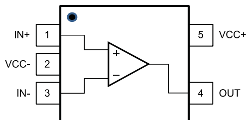
SOT23-5 (TSZ181)
