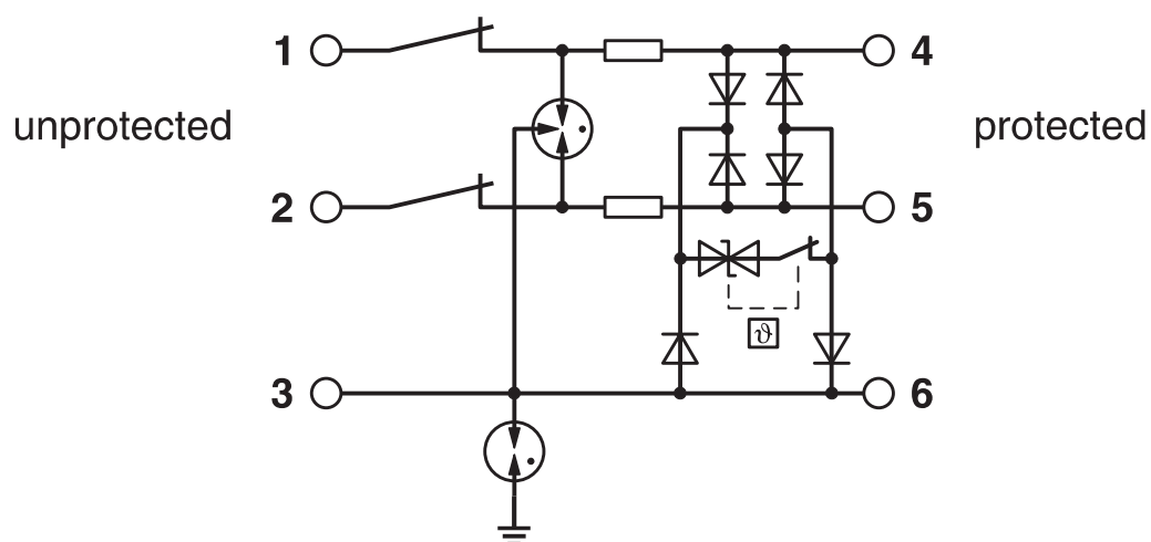
电路图
