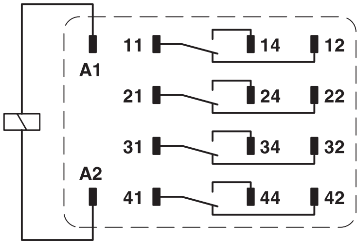
电路图
