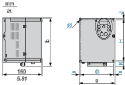
尺寸 (毫米)
