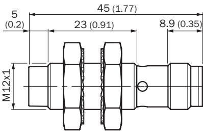
IMB12 短版, M12 插头, 非齐平
