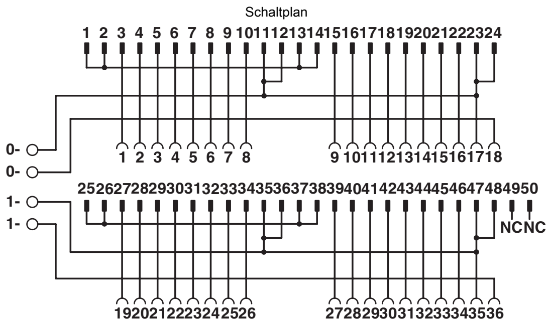
Anschlussbild FLKM 50-PA-AB/1756/IN/EXTC
