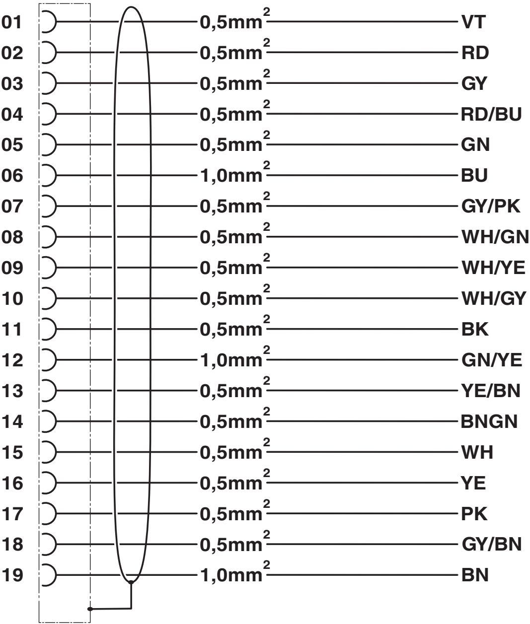
电路图
