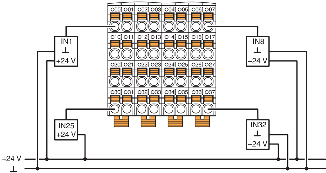
接线图
