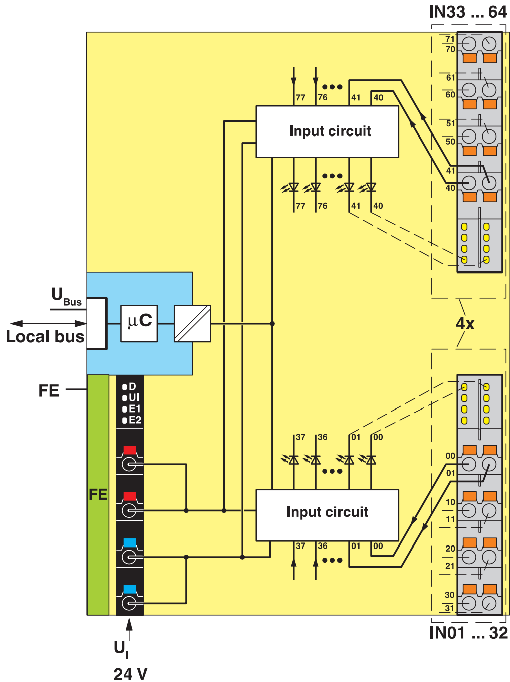
结构框图
