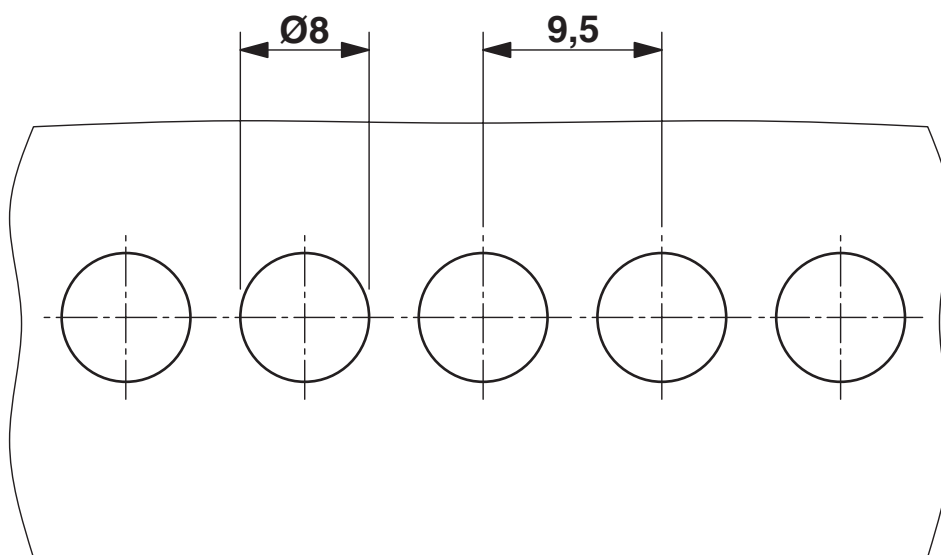
尺寸图
