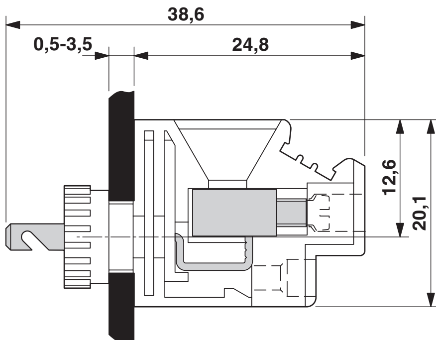
尺寸图
