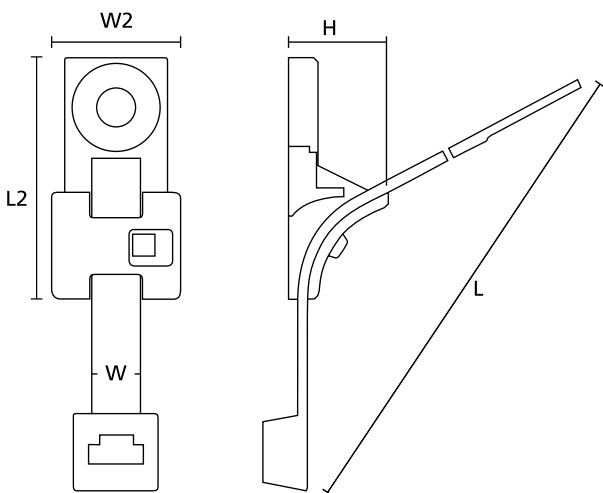
HDM con bridas (L = Longitud de la brida en "plano")
