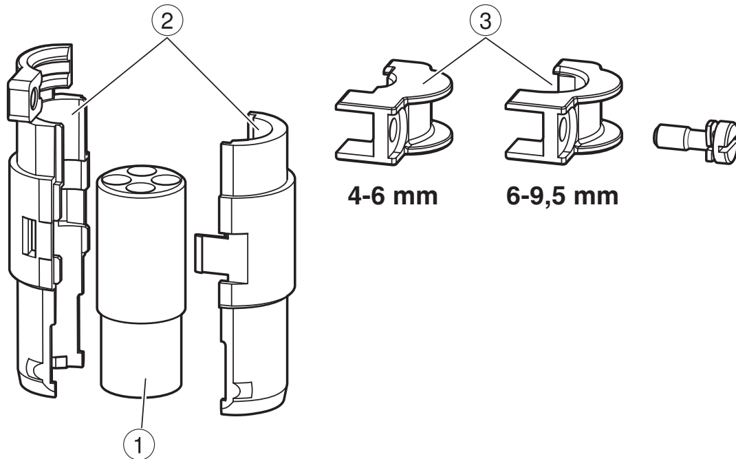
Funktionszeichnung
