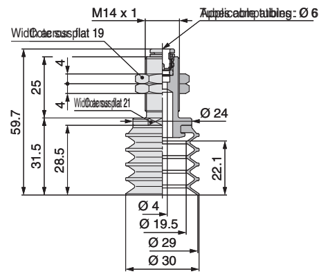
ZP2-TB30ZJS□-AL14-06
