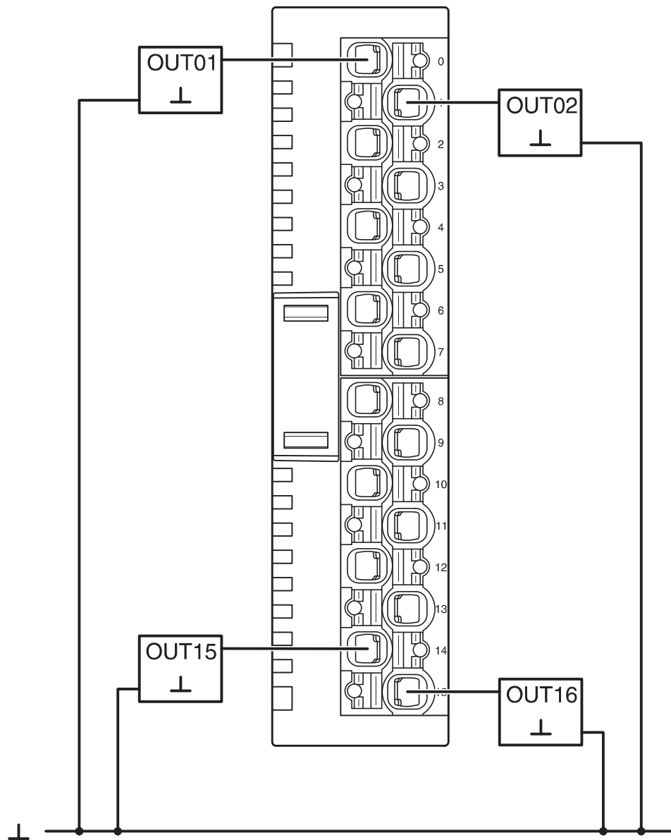
接线图
