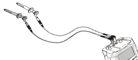
Figure 43. Connexions fixes « Heavy Duty » pour des mesures en multimètre utilisant des pinces crocodiles industrielles
