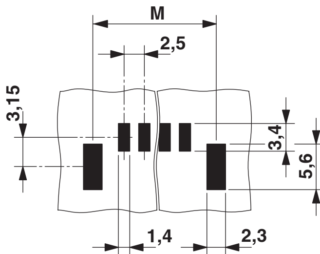
开孔图/焊盘环宽
