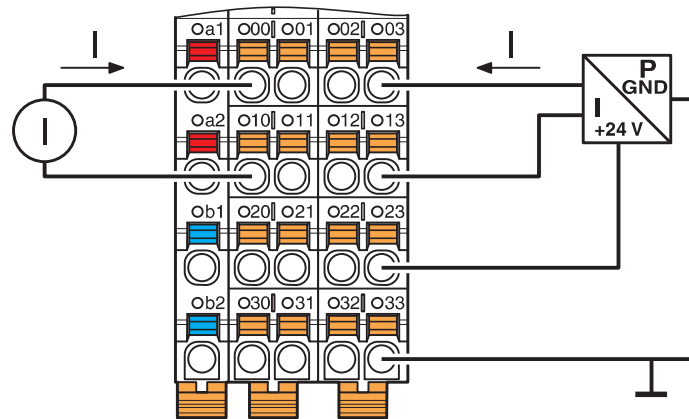
接线图
