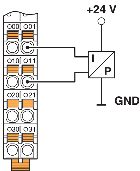
接线图
