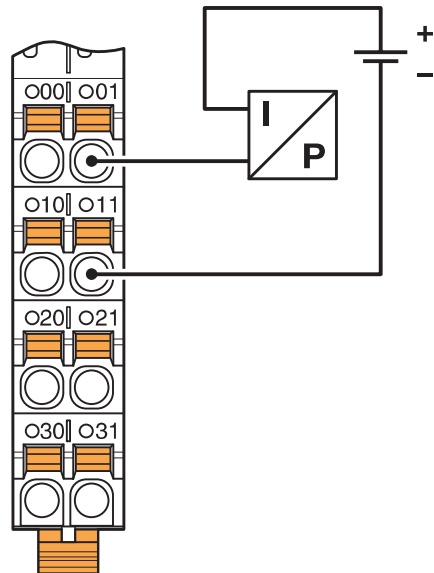
接线图
