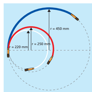
Overzicht van de buigradii van Cable Scout*
