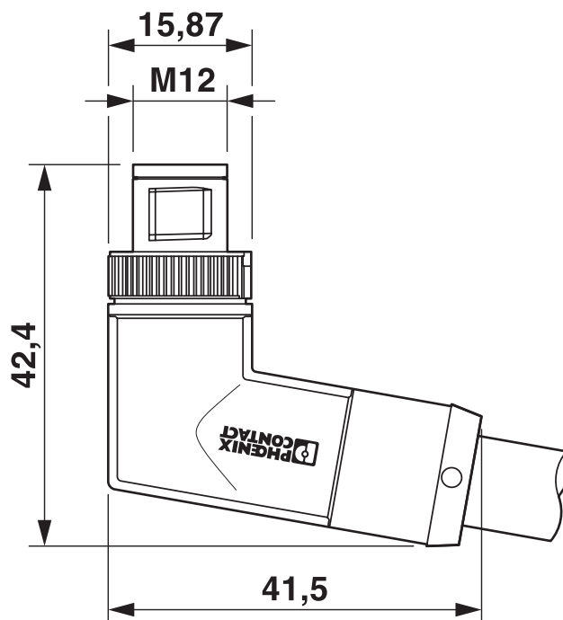
Maßzeichnung
