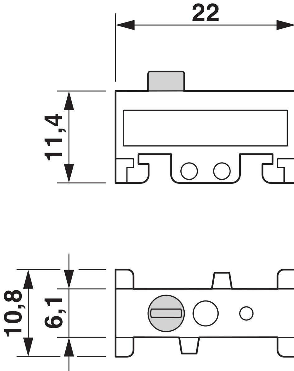
Maßzeichnung
