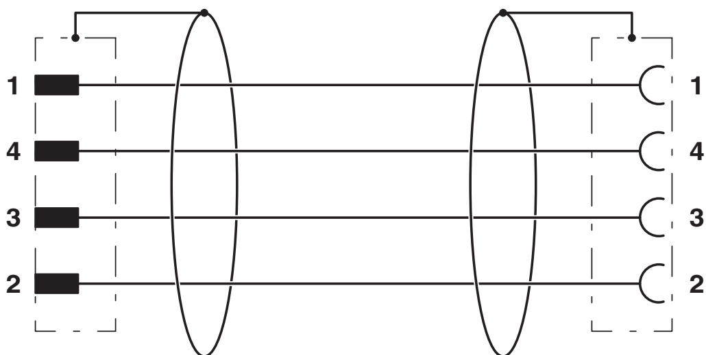
Kontaktbelegung der M8-Stecker / M12-Buchse
