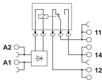
电路图
