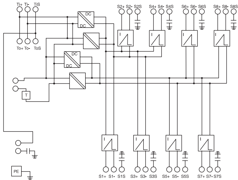
结构框图
