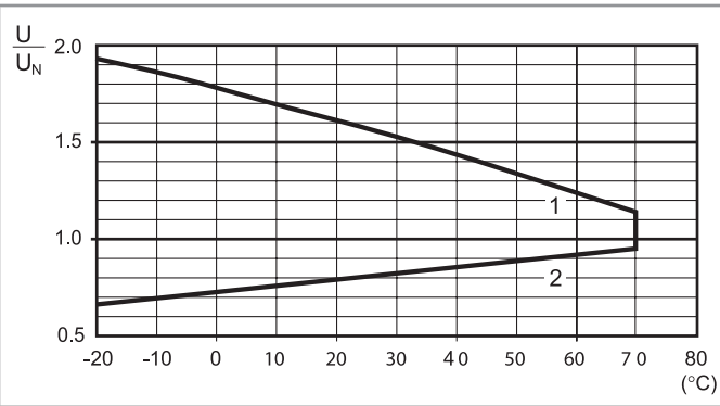
R 60 - Campo di funzionamento bobina DC in funzione della temperatura ambiente
