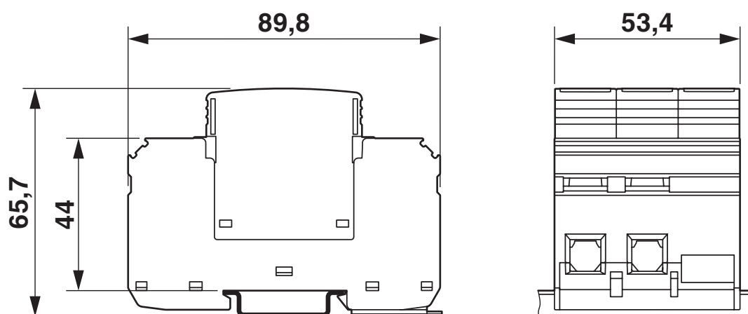
尺寸图
