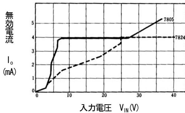
NJM7805/24 無効電流特性例 ( T_j=25^\circ\text{C} )
