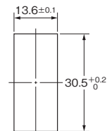
取り付け穴加工寸法 (BOTTOM VIEW)
