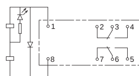
形G2R-2-SNDI(S) (DC仕様)
