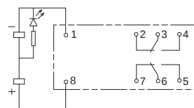
形G2R-2-SNI(S) (DC仕様)
