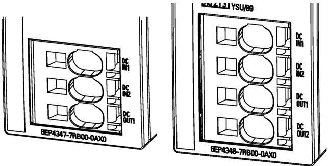
Bild 5: Eingang / Ausgang Figure 5: Input/output Figura 5: Entrada/salida 图 5: 输入，输出 Figure 5: Entrée/Sortie Figura 5: Ingresso / uscita Рисунок 5: Вход / выход Resim 5: Giriş / Çıkış
