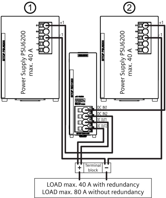
Bild 7: Verdrahtung 1 Modul (2 x 40 A) Figure 7: Wiring 1 module (2 x 40 A) Figura 7: Cableado 1 módulo (2 x 40 A) 图 7: 接线 1 模块 (2 x 40 A) Figure 7: Câblage 1 module (2 x 40 A) Figura 7: Cablaggio di 1 modulo (2 x 40 A) Рисунок 7: Электропроводка 1 модуля (2 x 40 A) Resim 7: 1 modülün kablolaması (2 x 40 A)
