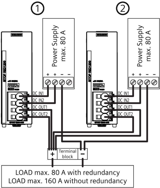
Bild 8: Verdrahtung 2 Module (2 x 20 A) Figure 8: Wiring 2 modules (2 x 20 A) Figura 8: Cableado 2 módulos (2 x 20 A) 图 8: 接线 2 模块 (2 x 20 A) Figure 8: Câblage 2 modules (2 x 20 A) Figura 8: Cablaggio di 2 moduli (2 x 20 A) Рисунок 8: Электропроводка 2 модулей (2 x 20 A) Resim 8: 2 modülün kablolaması (2 x 20 A)
