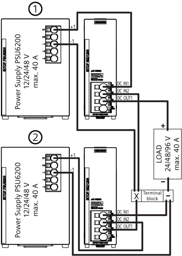
Bild 10: Reihenschaltung zur Spannungserhöhung 2 Figure 10: Series connection for increased voltage 2 Figura 10: Conexión en serie para aumentar la tensión 2 图 10: 为提高电压进行串联 2 Figure 10: Montage en série pour augmenter la tension 2 Figura 10: Collegamento in serie per aumentare la tensione 2 Рисунок 10: Последовательное подключение для повышения напряжения 2 Resim 10: Gerilim artırımı için seri devre 2
