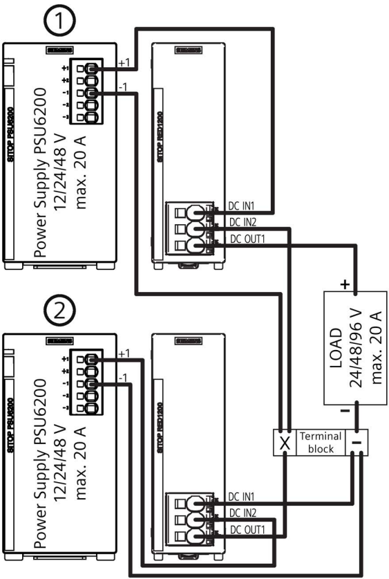
Bild 9: Reihenschaltung zur Spannungserhöhung 1 Figure 9: Series connection for increased voltage 1 Figura 9: Conexión en serie para aumentar la tensión 1 图 9: 为提高电压进行串联 1 Figure 9: Montage en série pour augmenter la tension 1 Figura 9: Collegamento in serie per aumentare la tensione 1 Рисунок 9: Последовательное подключение для повышения напряжения 1 Resim 9: Gerilim artırımı için seri devre 1
