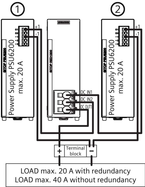
Bild 6: Verdrahtung 1 Modul (2 x 20 A) Figure 6: Wiring 1 module (2 x 20 A) Figura 6: Cableado 1 módulo (2 x 20 A) 图 6: 接线 1 模块 (2 x 20 A) Figure 6: Câblage 1 module (2 x 20 A) Figura 6: Cablaggio di 1 modulo (2 x 20 A) Рисунок 6: Электропроводка 1 модуля (2 x 20 А) Resim 6: 1 modülün kablolaması (2 x 20 A)
