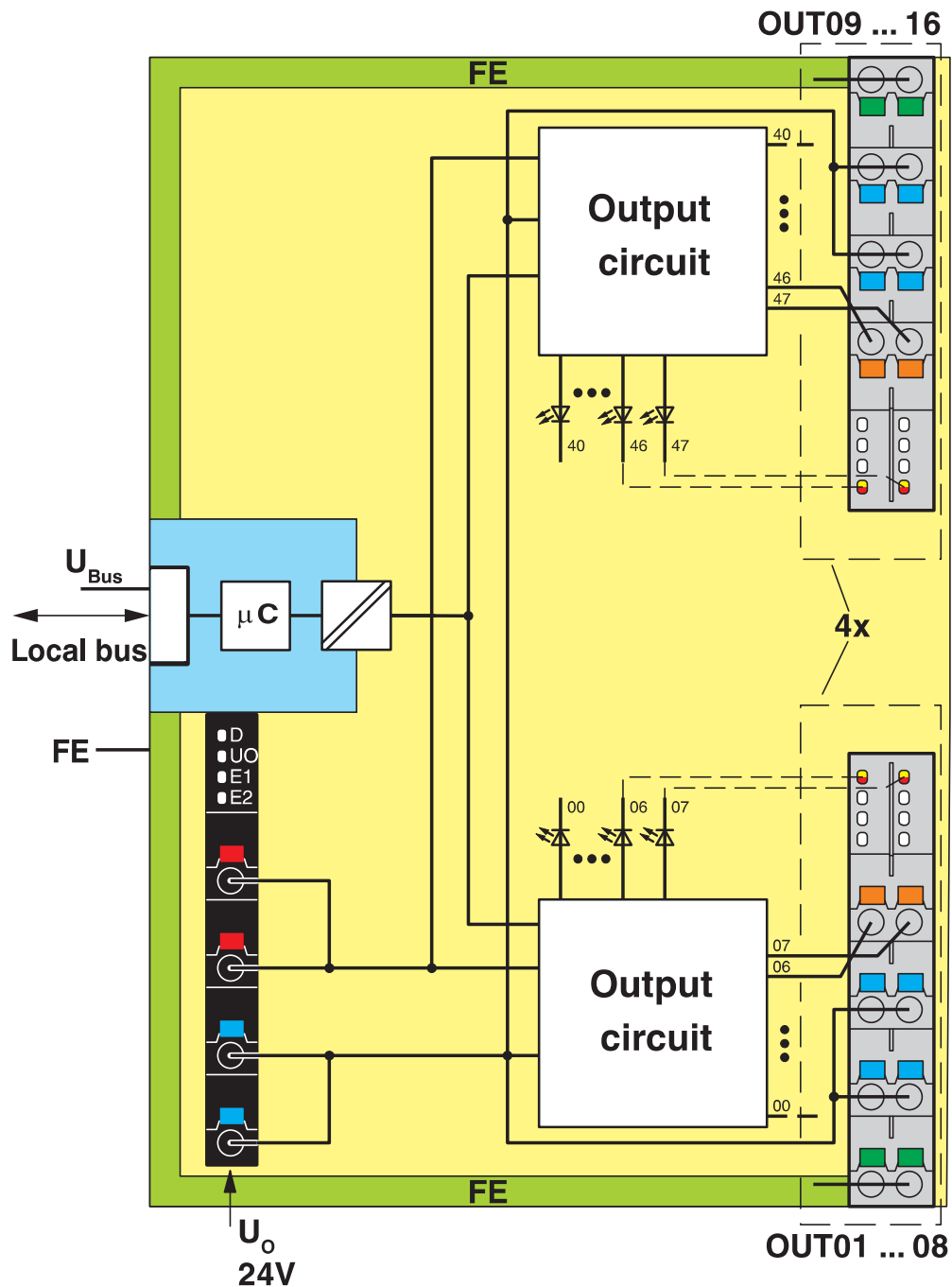
结构框图
