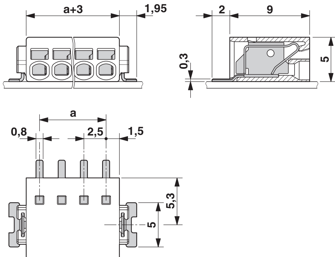
尺寸图
