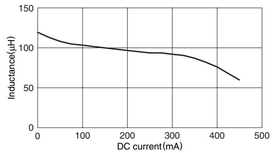
VLF5014AT-101MR26
