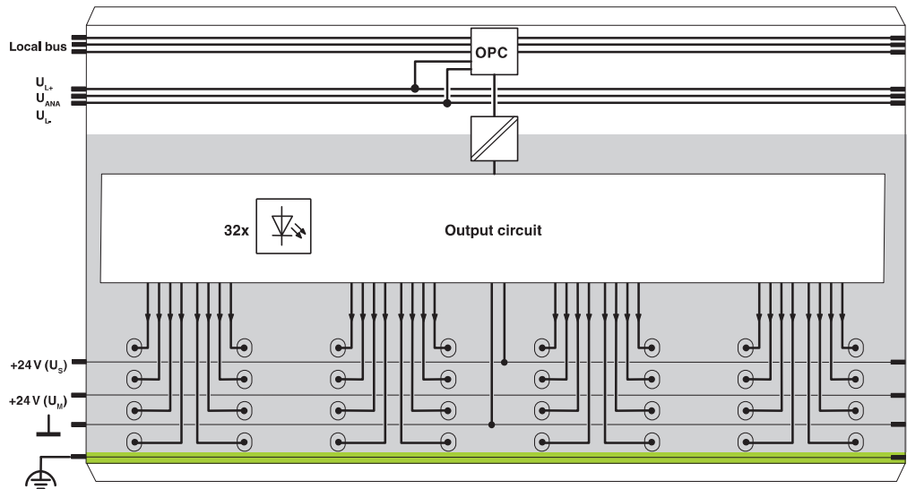
结构框图
