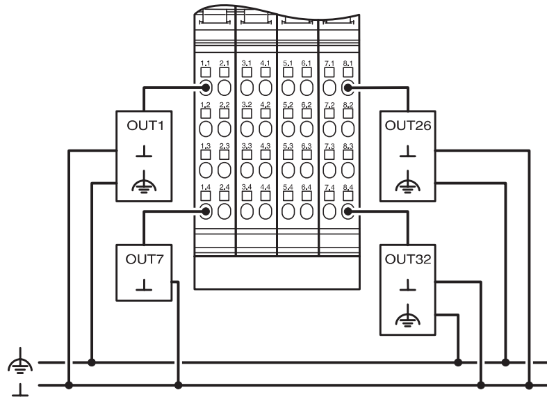
接线图
