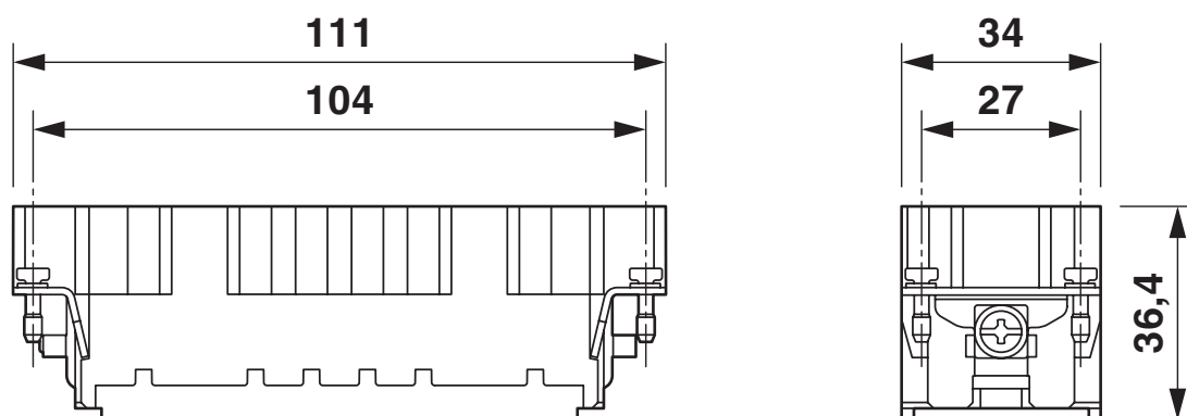
尺寸图
