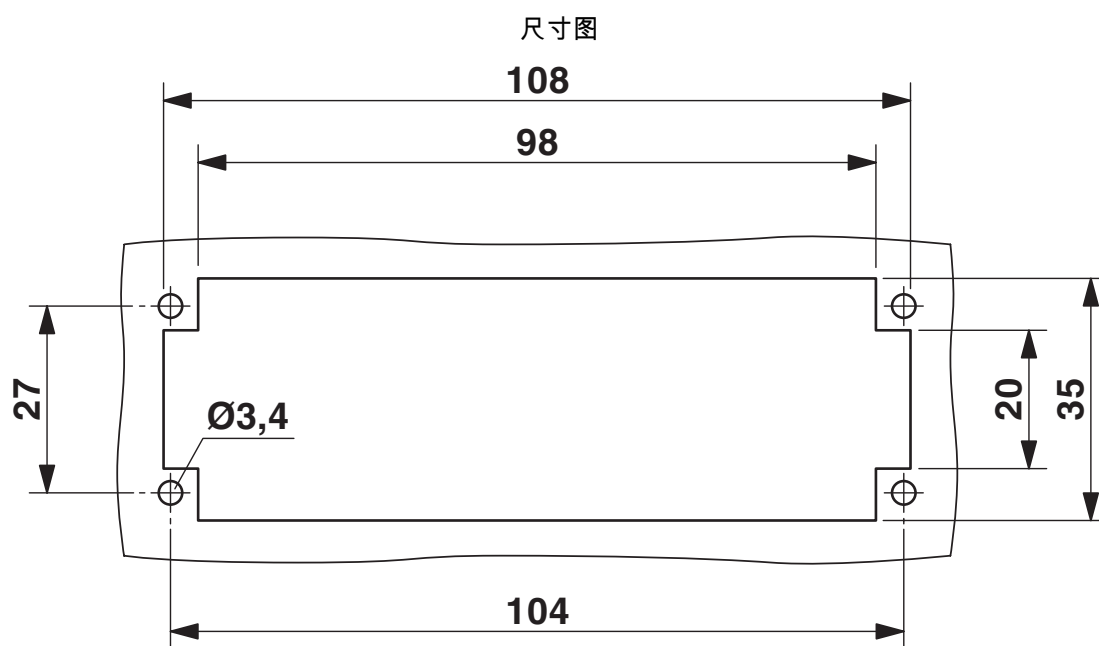
不使用外壳时的安装开口
