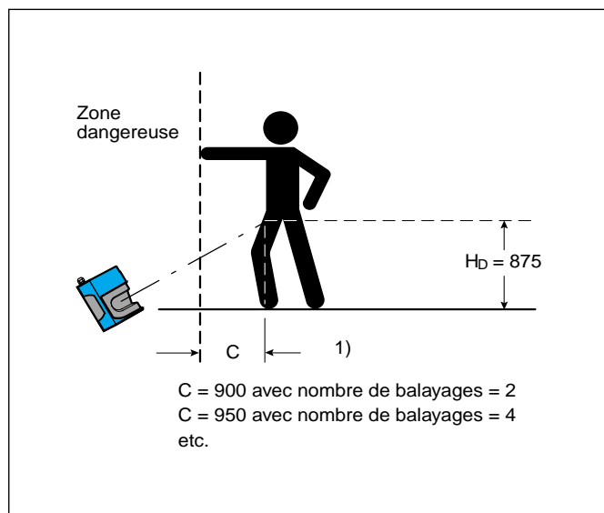
Cas 2b : bord du champ de protection à la hauteur maximale ( H_D = 875 )
