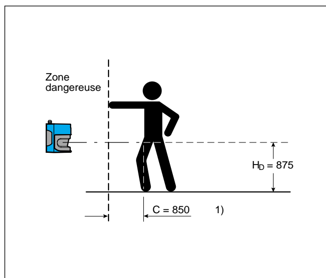
Cas 2a : bord du champ de protection à la hauteur maximale ( H_D = 875 )
