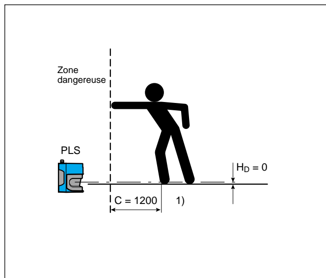
Cas 1 : bord du champ de protection au niveau du sol ( H_D = 0 )
