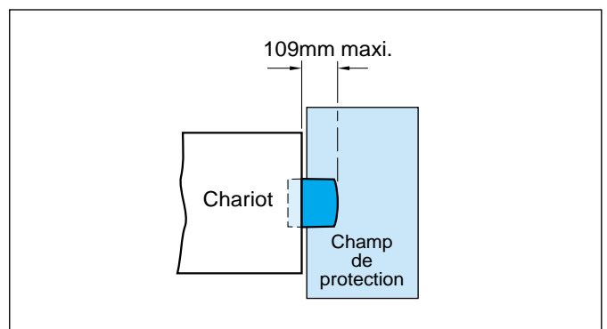
Type d'implantation. dans la carrosserie du chariot :
