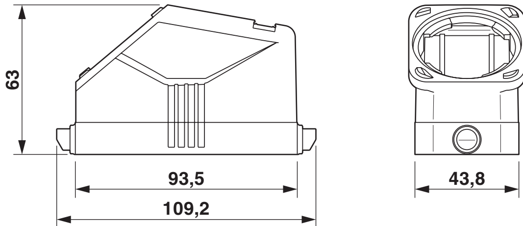
尺寸图
