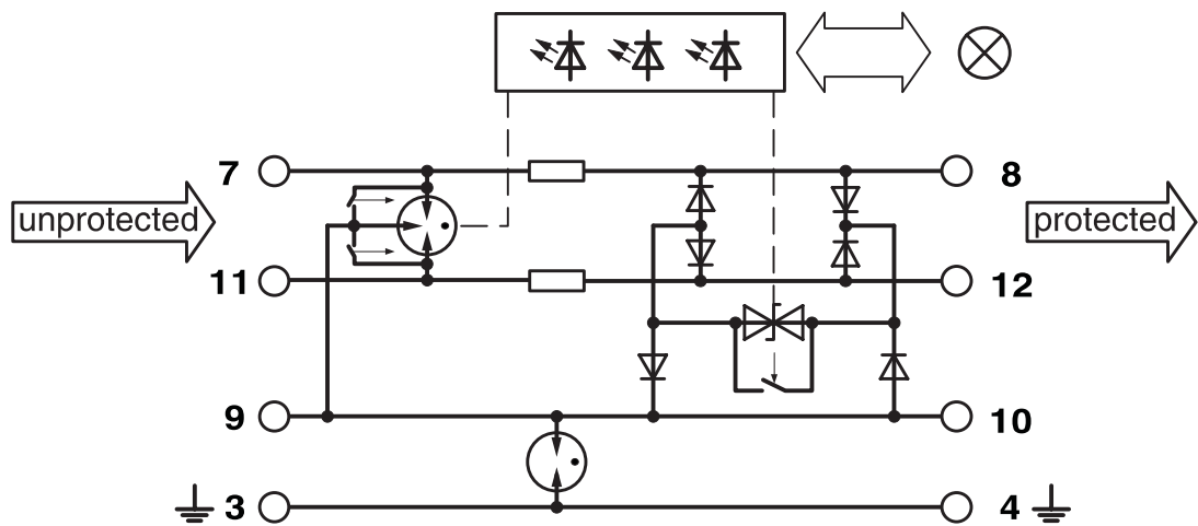
电路图
