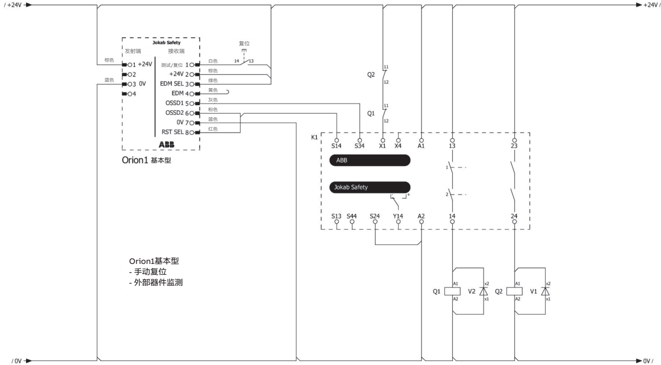
Orion1 基本型与 RT9 连接示例:
