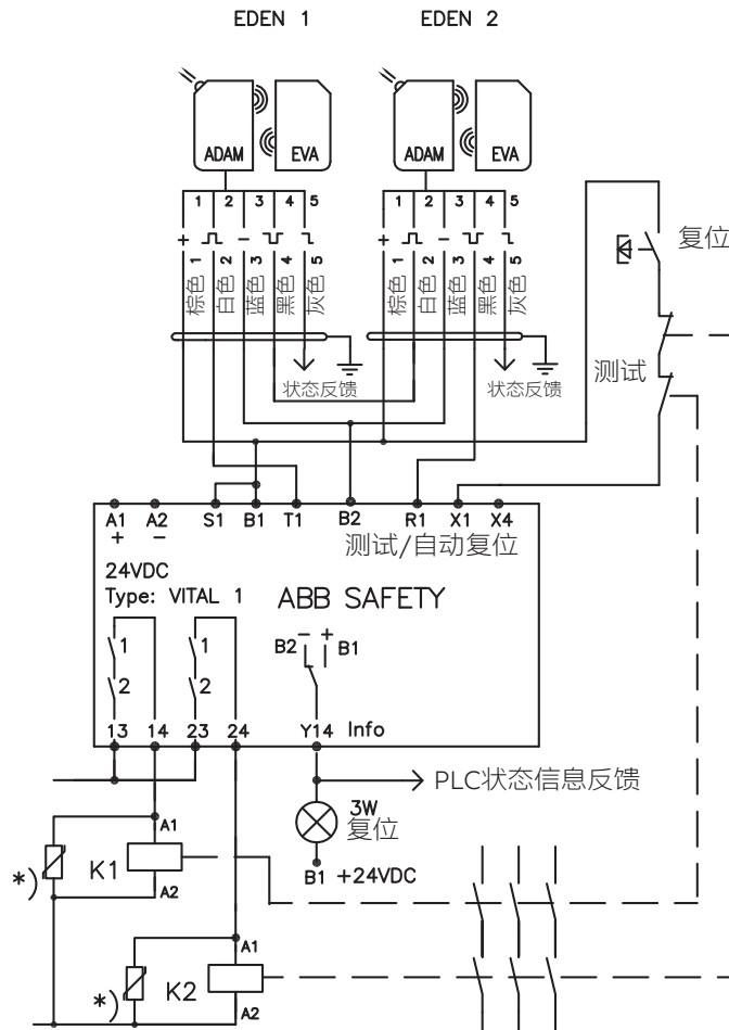
Eden DYN 与 Vital 连接示例
