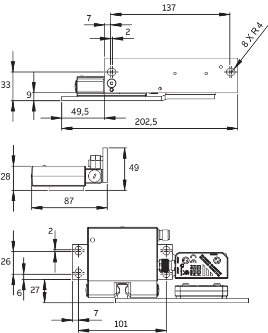
外形尺寸（mm） Dalton M12
