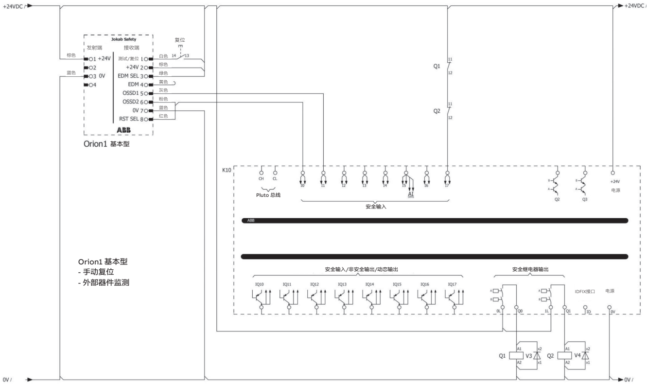
Orion1 基本型与 Pluto 连接示例:
