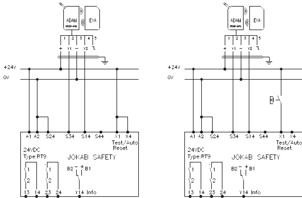
Eden OSSD 与 RT9 连接示例
