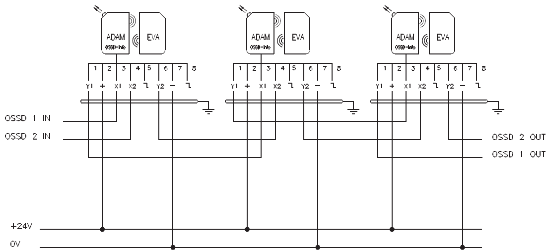
多个 Eden-OSSD 连接示例
