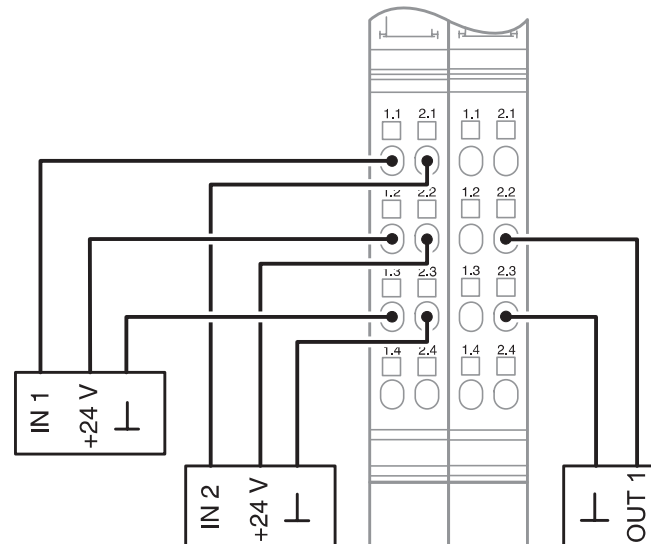
接线图
