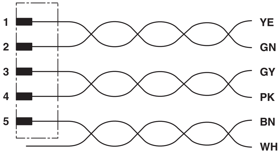
电路图
