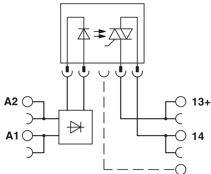
电路图
