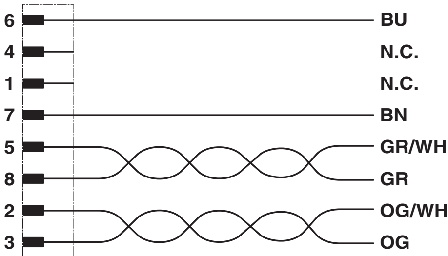
电路图
