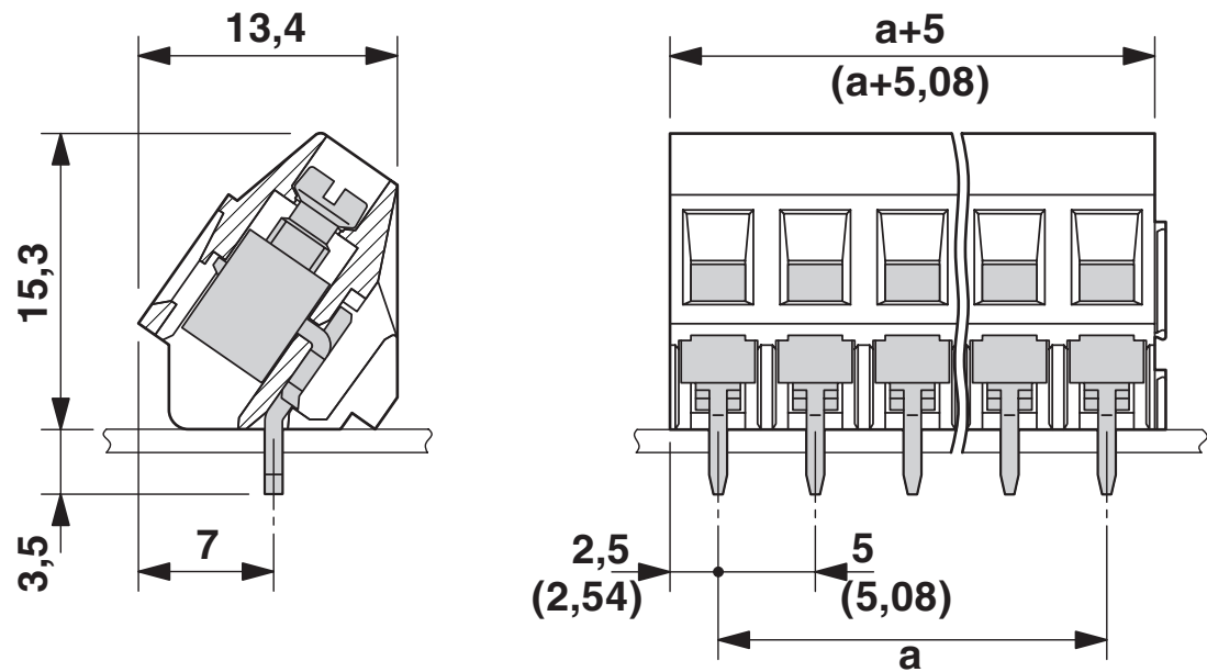
尺寸图
