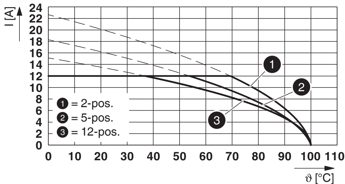
Typ: FKCT 2,5/...-ST mit MDSTBW 2,5/...-G
