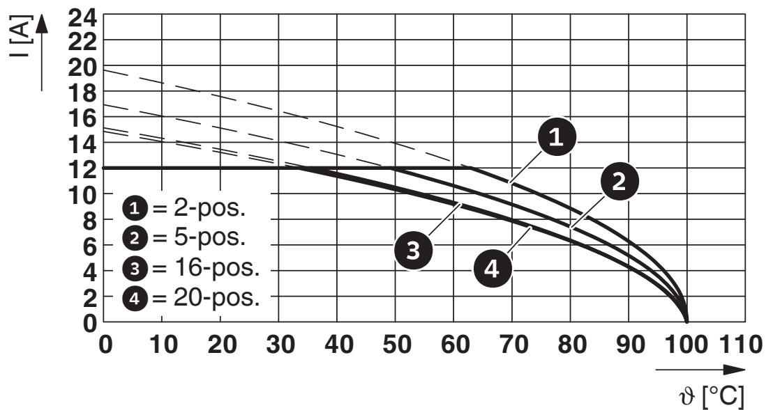
Typ: FKCT 2,5/...-ST mit MSTBVA 2,5/...-G
