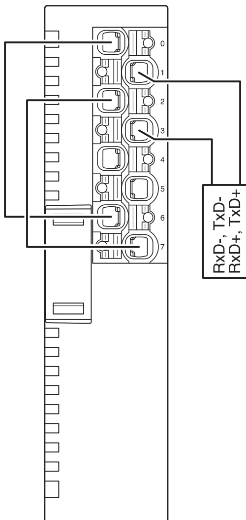
接线图
