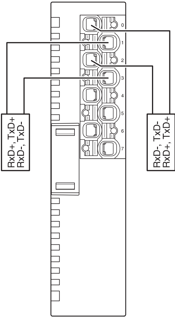
接线图
