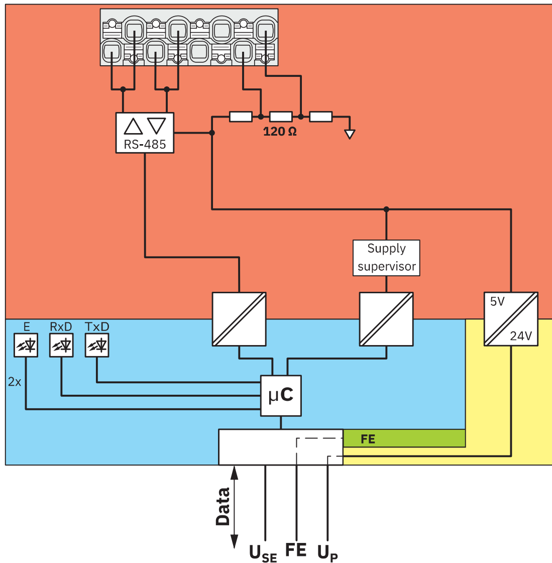
结构框图
