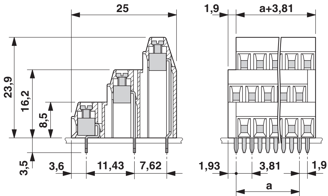
尺寸图
