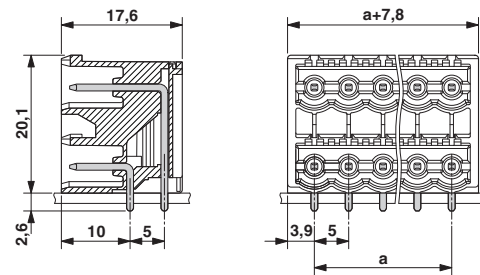
外形寸法
