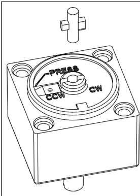
图 9.卡件与螺钉的分解图
