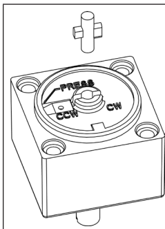
FIGURA 9. VISTA ESPLOSA DI MORSETTO E VITE
