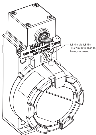
ABBILDUNG 10: ANWEISUNGEN ZUR VERDRAHTUNG
