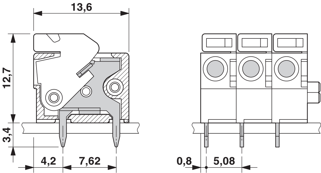
尺寸图
