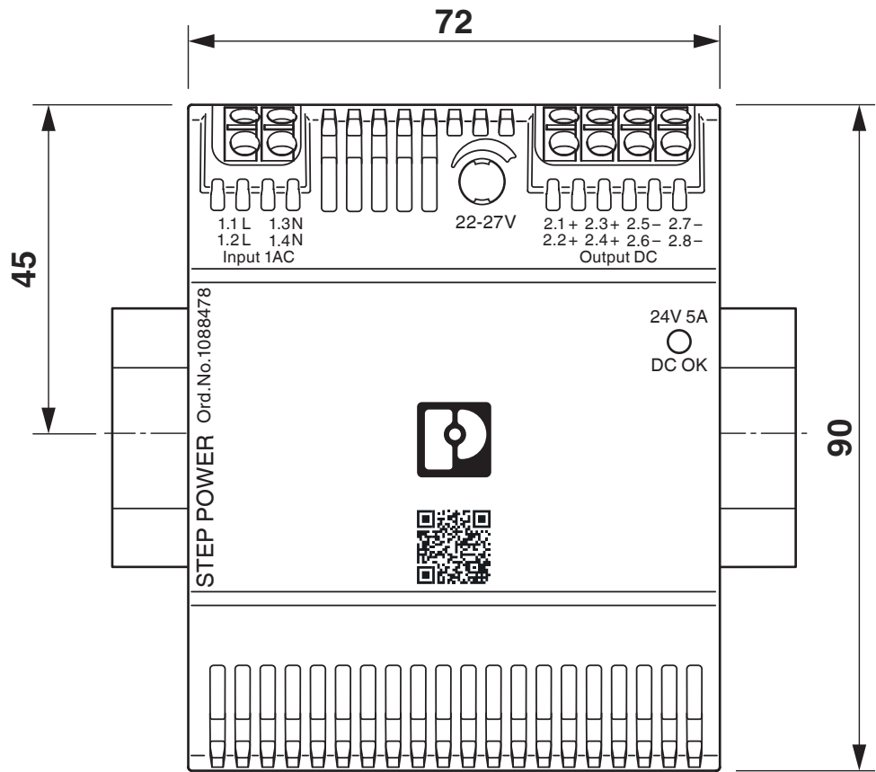
尺寸图
